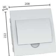
Dimensões da Base: 184x198x56mm
